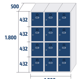
ECOC-40/3 PRO COD: 47070 65,1kg · 1,08m 3
