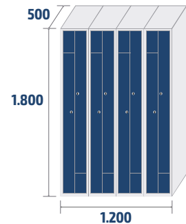
ECOL-30/4 PRO COD: 35304 79,8kg · 1,08m 3
