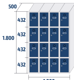
ECOC-30/4 PRO COD: 47066 71,2kg · 1,08m 3
