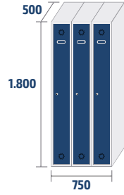
ECOV-25/3 PRO COD: 47002 39,1kg · 0,67m 3
