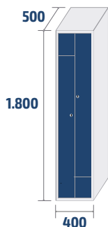
ECOL-40/1 PRO COD: 35401 28,1kg · 0,36m 3
