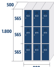
ECOM-30/3 PRO COD: 47048 51,6kg · 0,81m 3
